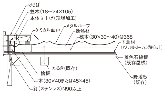
けらば部(けらば)
