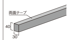
ケミカル面戸40谷 K40
